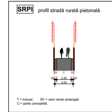
T = trotuar; SV = sant verde amenajat; C = parte carosabilă.
